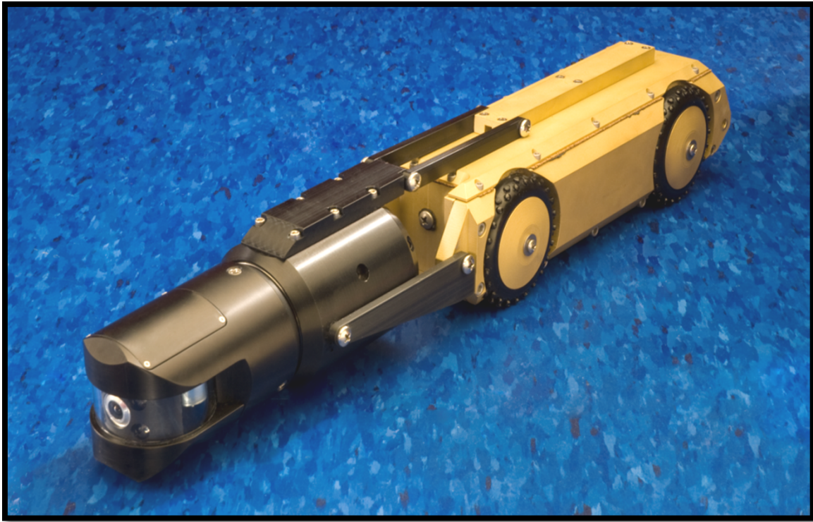
SHOWN WITH PROBE PAN & TILT MINI CAMERA
